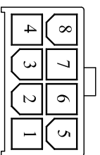
2x04P
